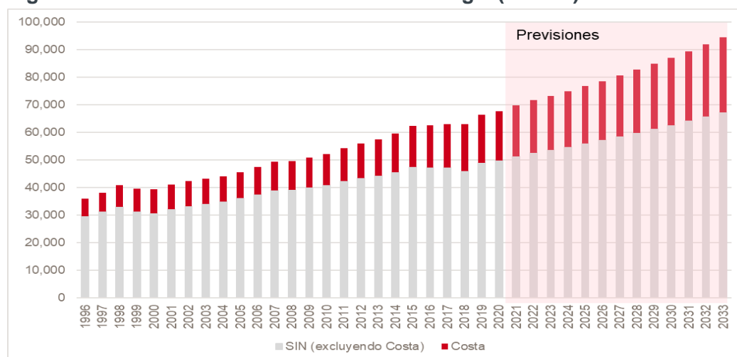
Figura 15 Evolución de la Demanda de energía (GWh-d)
