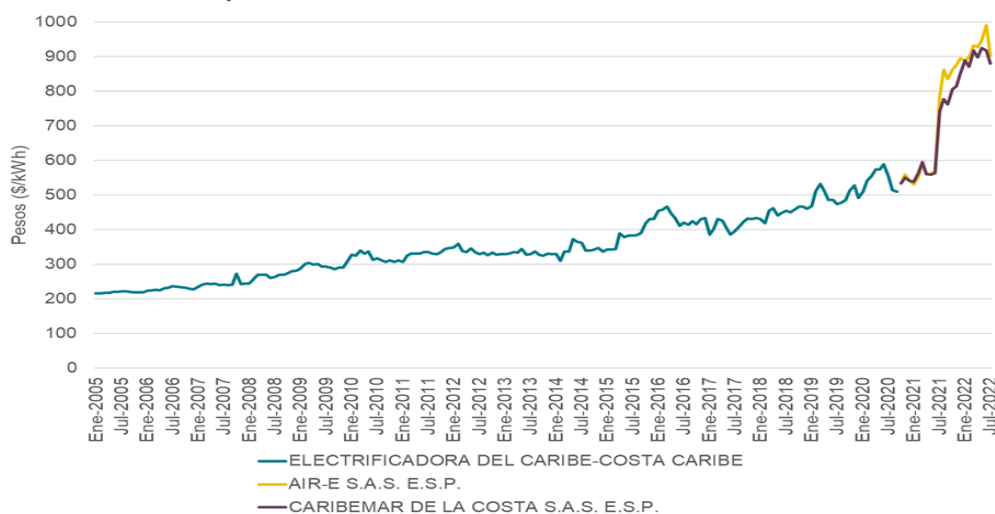
Figura 2 Evolución del CU en la región Caribe ($/kWh) (enero 2005- julio 2022)
