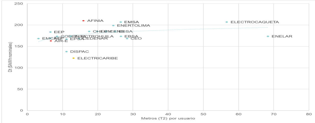
Figura 13 Cargo de distribución y metros de red (nivel 2) por usuario
