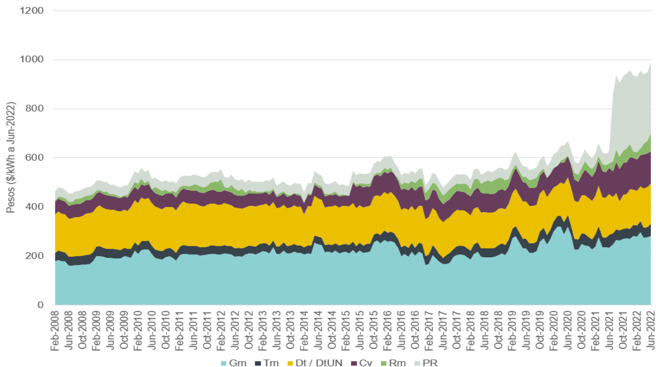
Figura 6 Componentes del Costo Unitario (CU) de Prestación del Servicio, a pesos de junio de 2022, Electricaribe y Air-e (febrero 2008-junio 2022)
