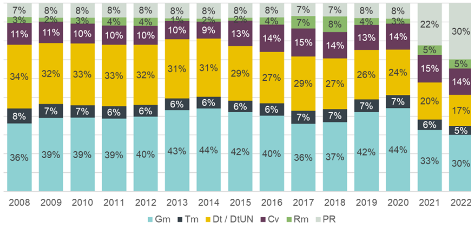
Figura 4 Composición del CU: Electricaribe (2008-2020) Y Air-e (2020-2022)
