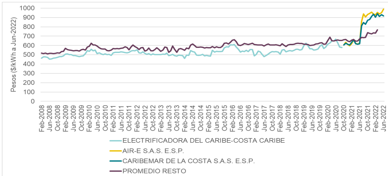
Figura 12 Costo Unitario (CU) de Prestación del Servicio, a pesos de junio de 2022 (febrero 2008-junio 2022)
