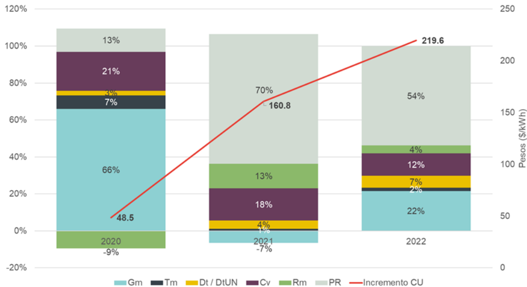
Figura 8 Contribución en los cambios del CU. Air-e (2020-2022)
